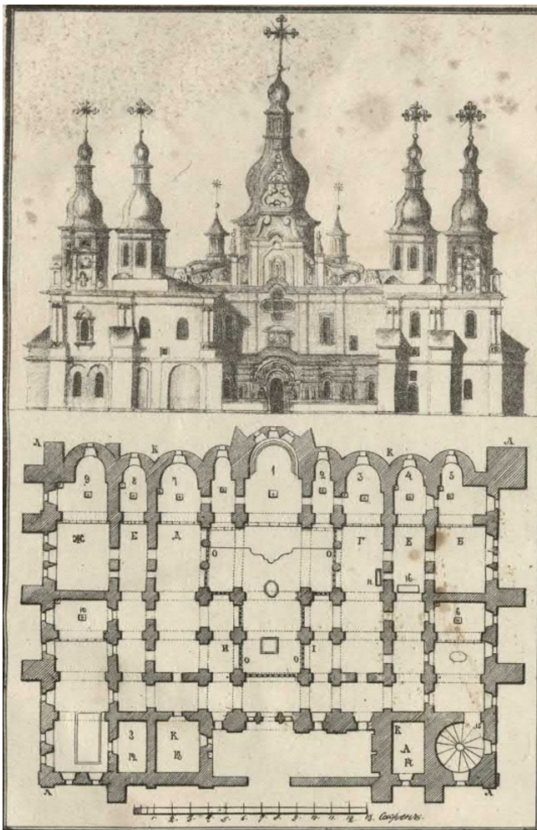
План и фасад Софийского собора в Киеве
